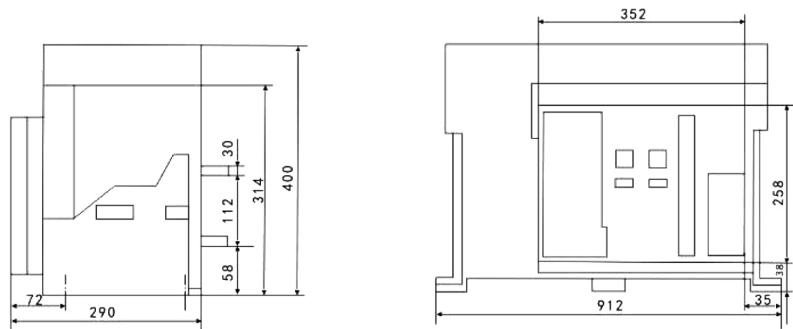
水平端子接线
