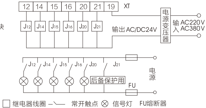
断路器附加功能用继电器接线图
