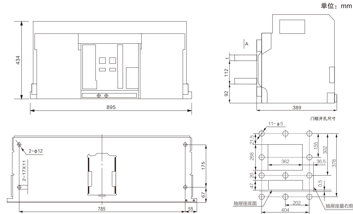
用户连接铜排规格、数量
