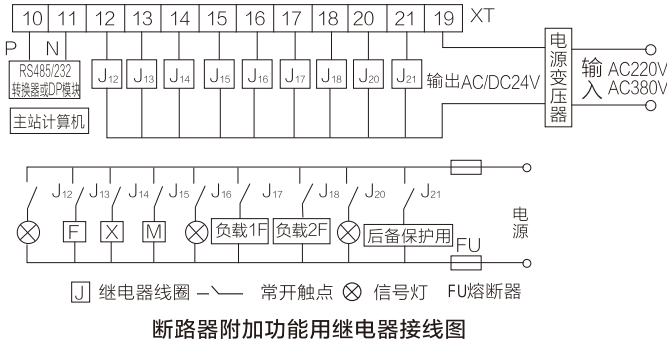
断路器附加功能用继电器接线图
