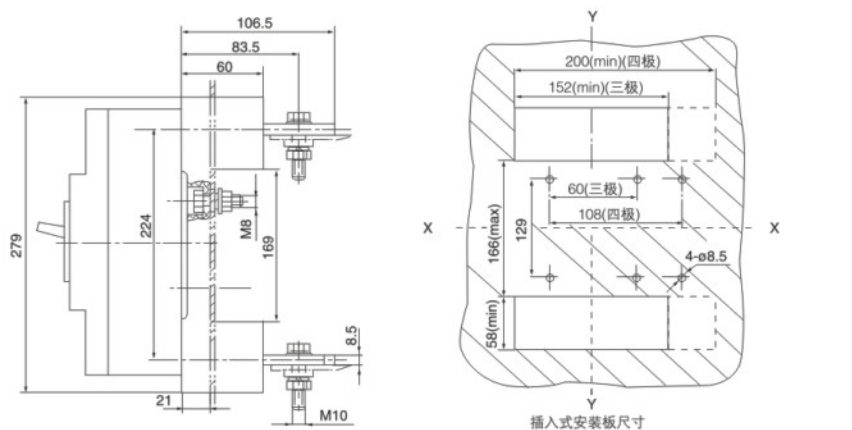
□ HTM1-400(L、M、H)，HTM1L-400(M、H)插入式(三极、四极) X-X、Y-Y为三极断路器中心
