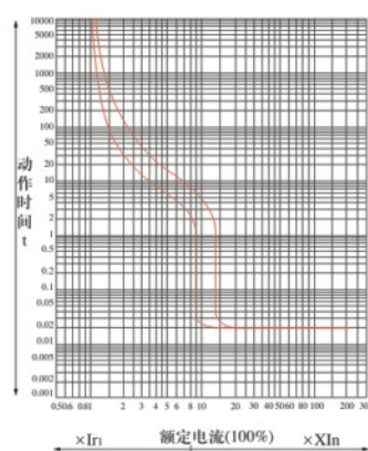
HTM1-100L、M、H时间/电流特性曲线
