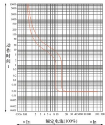
HTM1-225L、M、H时间/电流特性曲线
