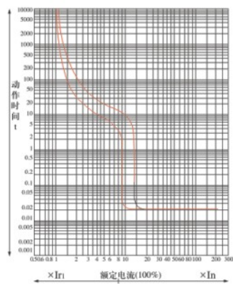
HTM1-400L、M、H时间/电流特性曲线
