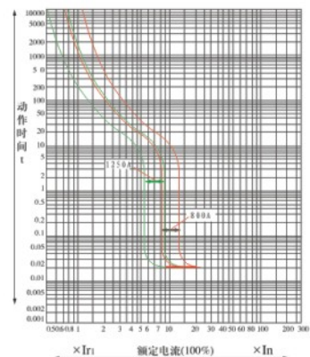
HTM1-800、1250M、H时间/电流特性曲线
