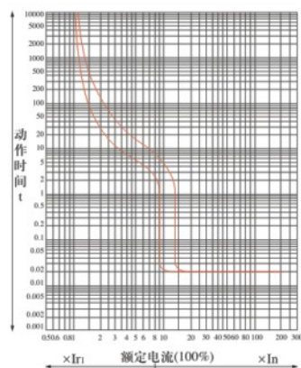
HTM1-63L、M时间/电流特性曲线
