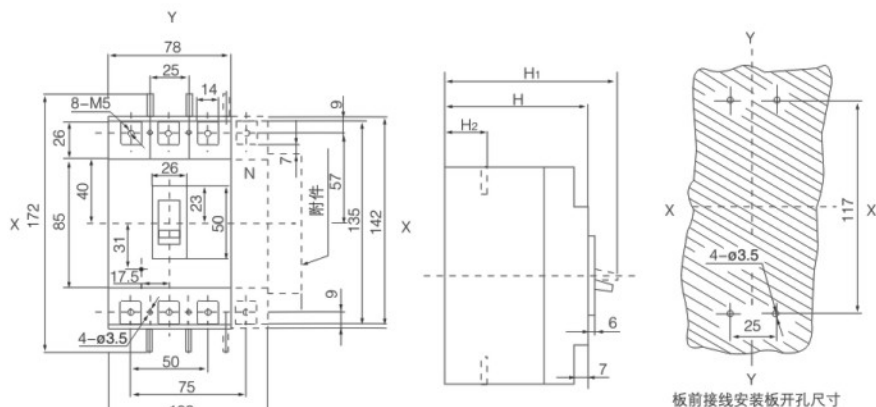
□ HTM1-63(L、M)板前接线(三极、四极) X-X、Y-Y为三极断路器中心
