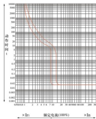
HTM1-630L、M、H时间/电流特性曲线
